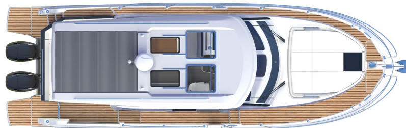
TOP VIEW WITH OPENING ROOF PLAN DE PONT AVEC TOIT OUVRANT
