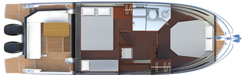
LOWER DECK PONT INFÉRIEUR
